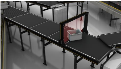
Bild 2: Die neue Generation von Interroll-Einschussförderern (sogenannte Infeeds).
